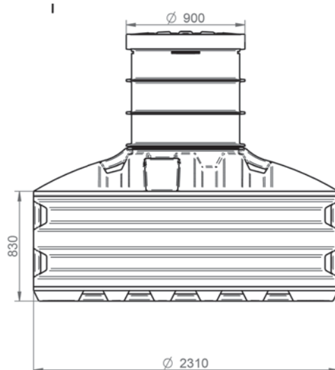
Flexibel anslutningsdimension
